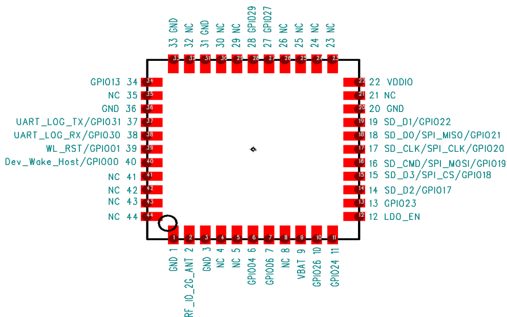
图 6-1 管脚排列
